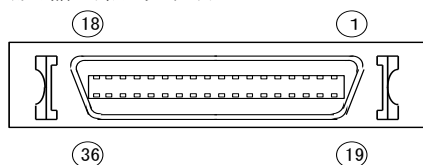
计数器侧插针配置图 (DX10M-36S)
